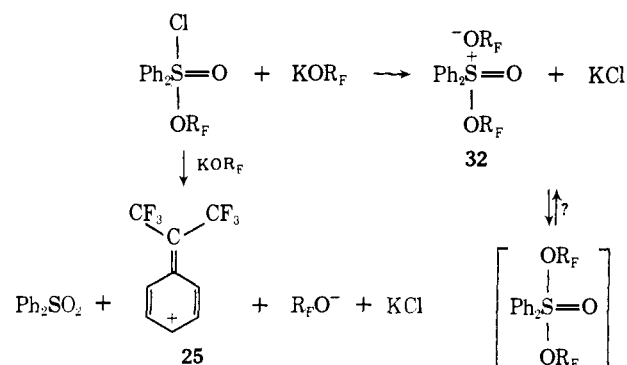
Scheme VI
